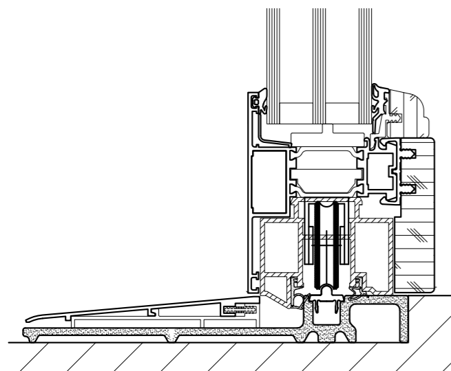
VITRASLIDE Alu-Holz-System-Konstruktion für Schiebeelemente. Sistema con struttura in alluminio e legno per elementi scorrevoli U_w \leq 0,7 \text{ W/m}^2 \text{ K}
