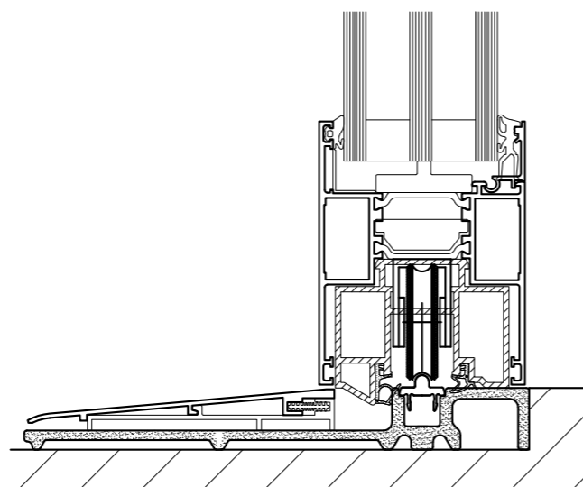
VITRASLIDE AL Alu-System-Konstruktion für Schiebeelemente. Sistema con struttura in alluminio per elementi scorrevoli U_w \leq 0,8 \text{ W/m}^2 \text{ K}
